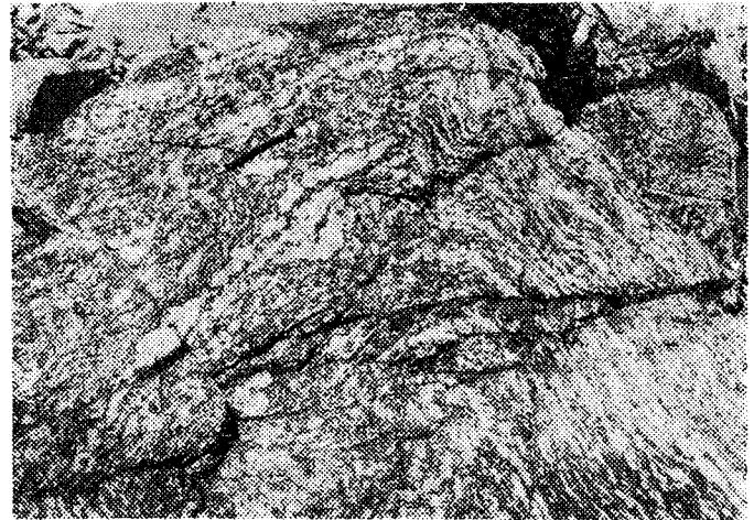
Şekil 5: Kıvrımlanmış bantlı migmatitler.
